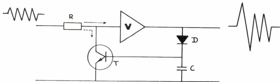
Fig. 6: Principe van automatische volumeregeling.
