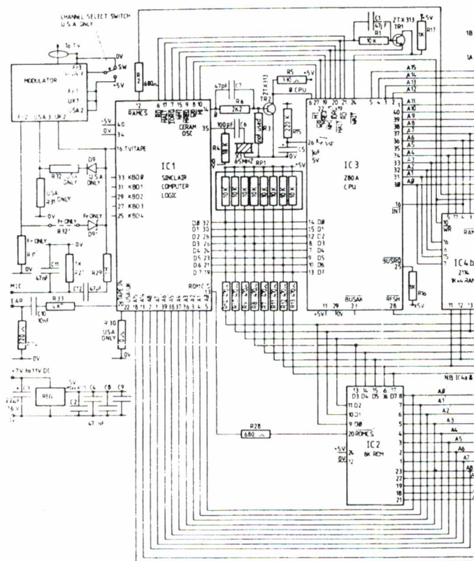
Fig. 2: Deelschema ZX 81
