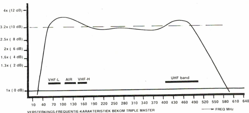
FIG. 1: VERSTERKINGSKARAKTERISTIEK BEKOM TRIPLE MASTER ANTENNEVERSTERKER GEMETEN OVER 6 EXEMPLAREN
