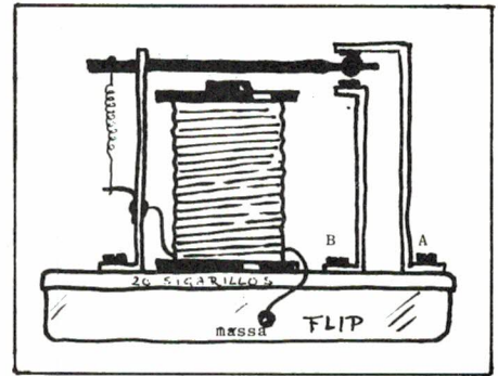
Fig. 2. De praktische uitvoering. Wie een beetje handig is kan ook het relais zelf maken door flink wat wikkelingen dun, geïsoleerd koperdraad op een zelfgemaakte klosje te wikkelen.
