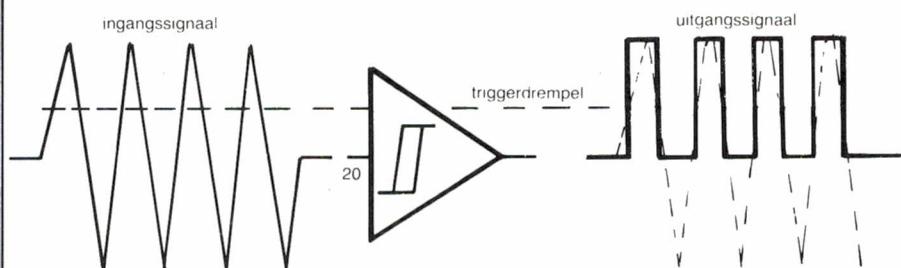
Fig. 5: De triggerschakeling in J = 1C 1 (pen 20) zet ingangssignalen die hoger zijn dan de trigger drempel om in blokgolven.
